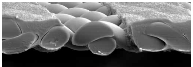
Απευθείας επάλειψη στη γάζα με EOM 4 μm σε SEFAR PET 1500 180-27Y
