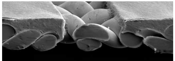
Capillary film 15μm με 7 μm EOM σε SEFAR PET 1500 180-27Y
