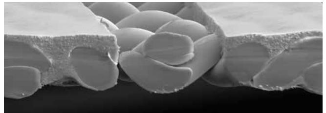
Τετράγωνισμένο κανάλι εκτύπωσης με SEFAR PCF FC 180-27Y, με συσσώρευση εμουλσιόν (eom) 3μm
